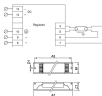
Technische Daten Philips HF-R 136 TL-D EII 220-240V für 1x36W
